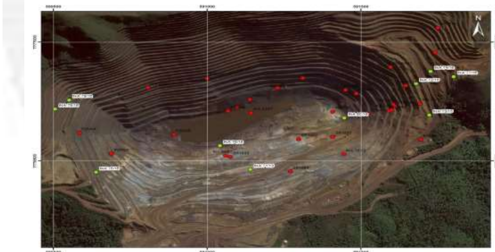
Figura 12: Localização dos instrumentos de monitoramento de nível d'água na mina Córrego do Feijão.
